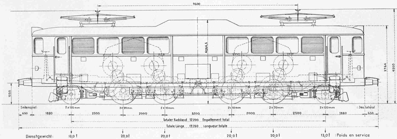
Abb. 9. A e 4/6 Schnell- und Güterzuglokomotive der SBB, gebaut 1941 durch SLM Winterthur, BBC, MFO und SAAS. — Typensklisse 1:100
