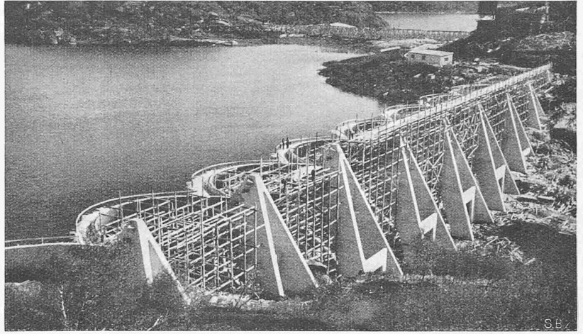
Abb. 8. Navanndamm des Vest Agder Elektrizitätswerks, im Bau
