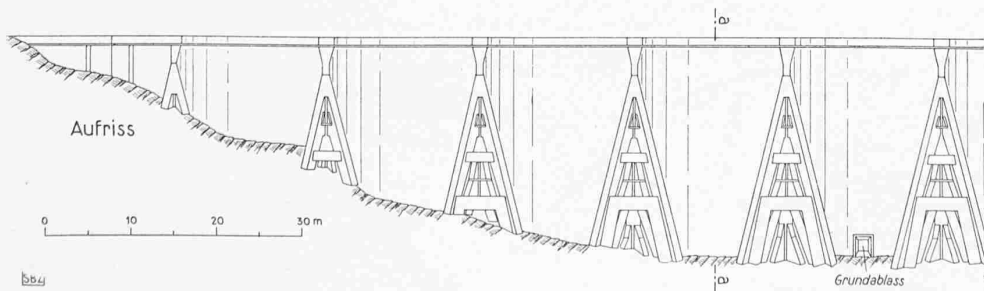
Abb. 10 u. 11. Navandamm, Teilgrundriss und luftseitige Ansicht 1:800
