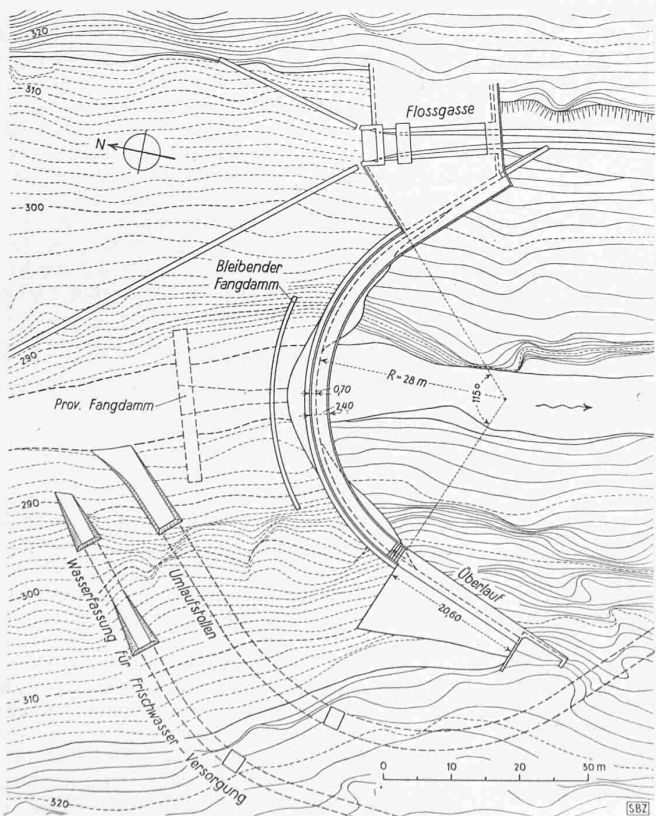
Abb. 13. Langliddamm-Bogenmauer, Lageplan 1:1000
