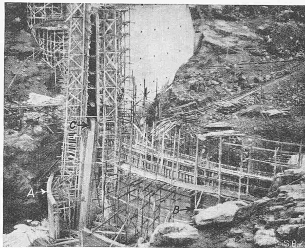
A (rechts) bleibender Fangdamm, B Schwindfuge, C horizontale Baufuge
