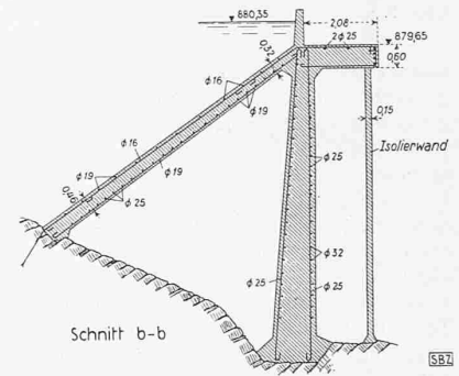
Abb. 17. Bjölsegrödam, Schnitt b-b 1:200
