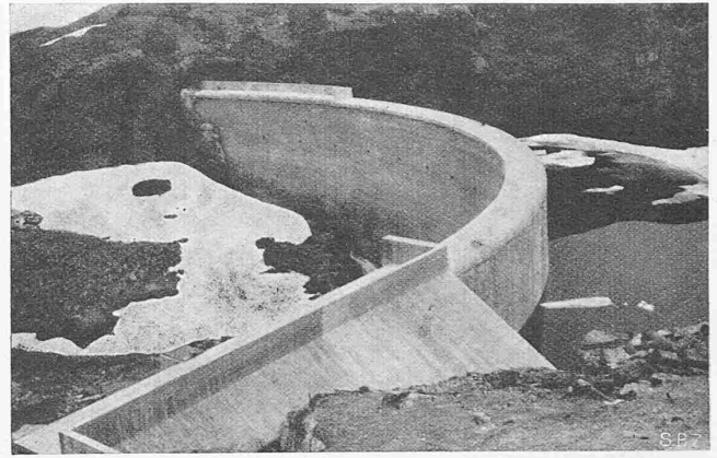
Abb. 14. Bjölsegrö-Bogenstaumauer
