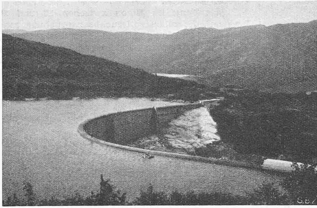
Abb. 22. Skjerkavann-Bogenstaumauer
