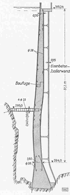
Abb. 19. Schnitt Masstab 1:400
