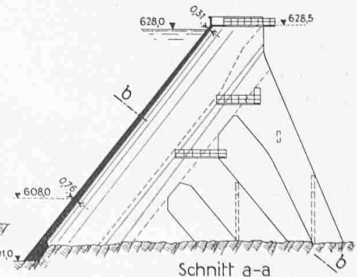
Abb. 12 u. 13. Schnitte 1:800
