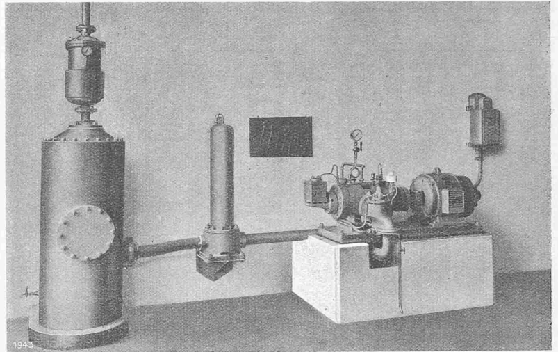
SLM Winterthur Druckluft-Kompressorenanlage mit Wasserschmierung
