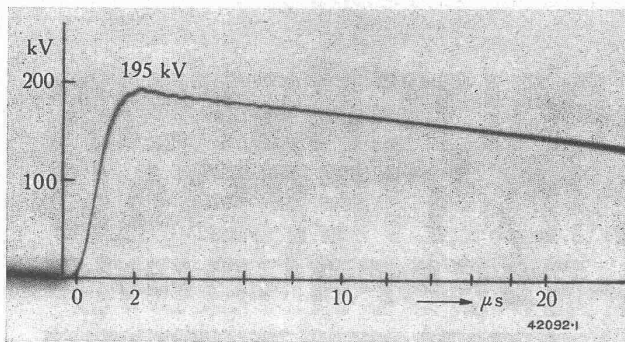
Verlauf des Spannungsstosses ohne Überspannungsableiter
