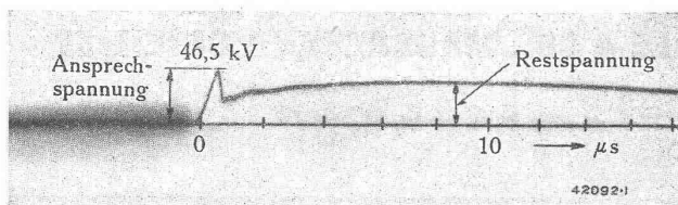
Verlauf des Spannungsstosses mit Überspannungsableiter
