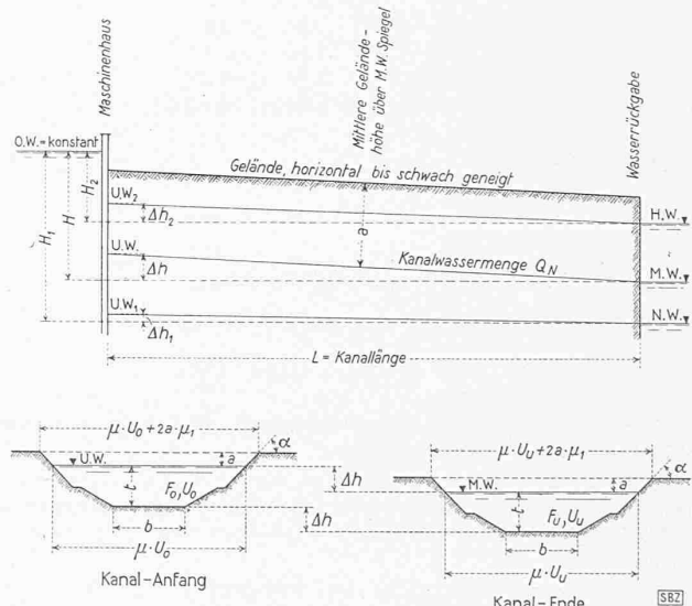
Abb. 2. Wasserspiegelbreite \mu U , wobei U_0 \cong U_0 ; \mu < 1 Geländebreite \mu U + 2\mu_1 a , wobei U_0 \cong U_0 ; \mu_1 > 1 = f(a)
