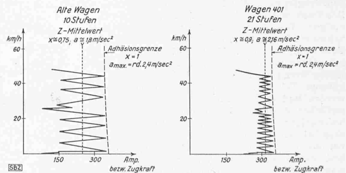
Abb. 11. Geschwindigkeit in Funktion der Zugkraft. Abhängigkeit des Ausnutzungsgrades x des Reibungskoeffizienten \mu von der Stufenzahl
