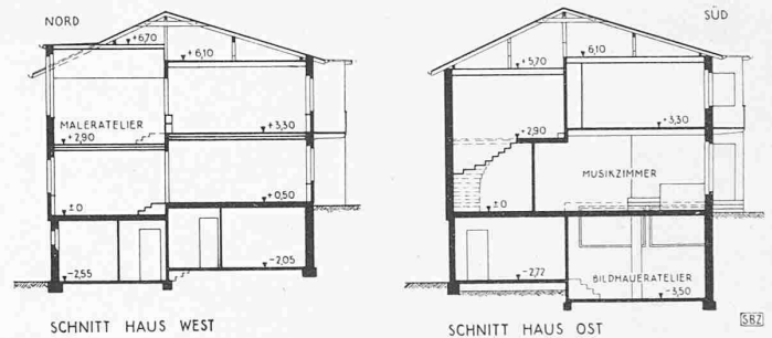
Abb. 8. Querschnitte senkrecht zur Dachfirst. — 1:300
