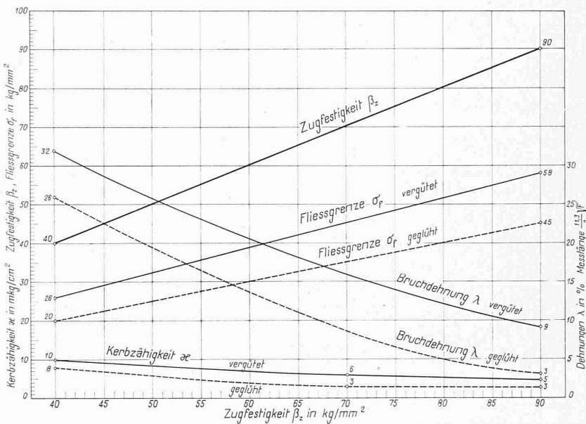
Abb. 7. Stahlguss. Zugfestigkeit, Streckgrenze, Bruchdehnung und Kerbzähigkeit. Hochwertige, legierte Stahlgussarten \beta_z \geq 70 kg/mm 2 weisen höhere Kerbzähigkeiten auf
