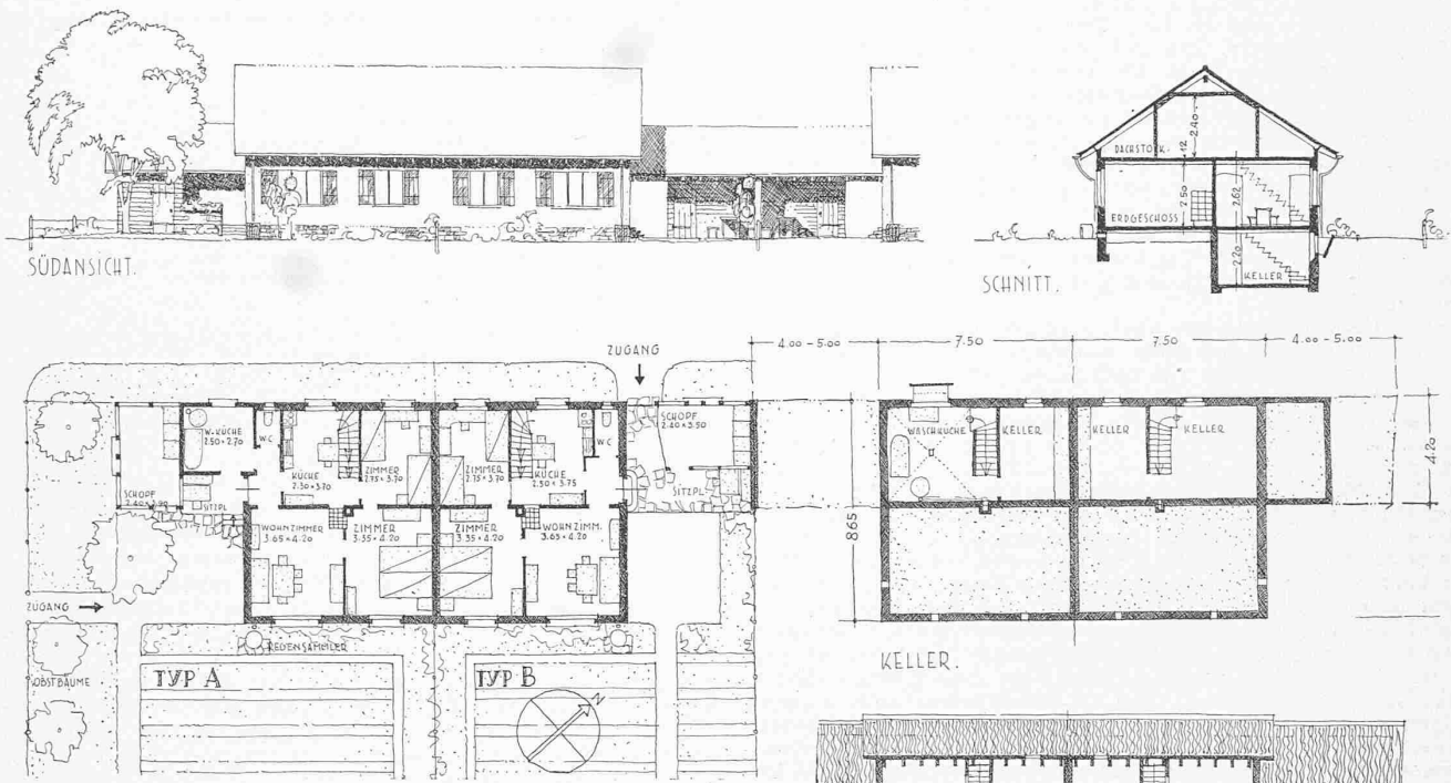
Grundrisse, Schnitt, Südansicht 1 : 300. Lageplan 1 : 3500
