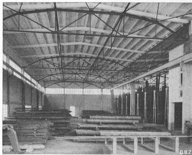
Abb. 6. Innenaussicht der Halle 1, rechts hinten Halle 2
