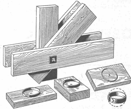
RINGDÜBEL \oplus PATENT Knotenpunktverbindung für hölzerne Tragwerke
