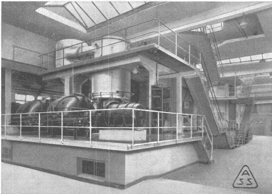
Von uns projektierte u. erstellte Eindampfanlage für Milch, Obstsaft etc. mit Wärmepumpe (Turbo-Verdichter)
