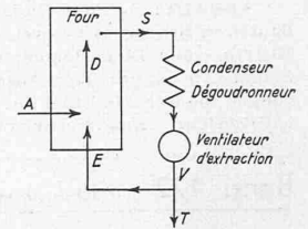
Fig. 2. Schéma de circulation des gaz dans le four ERIM
