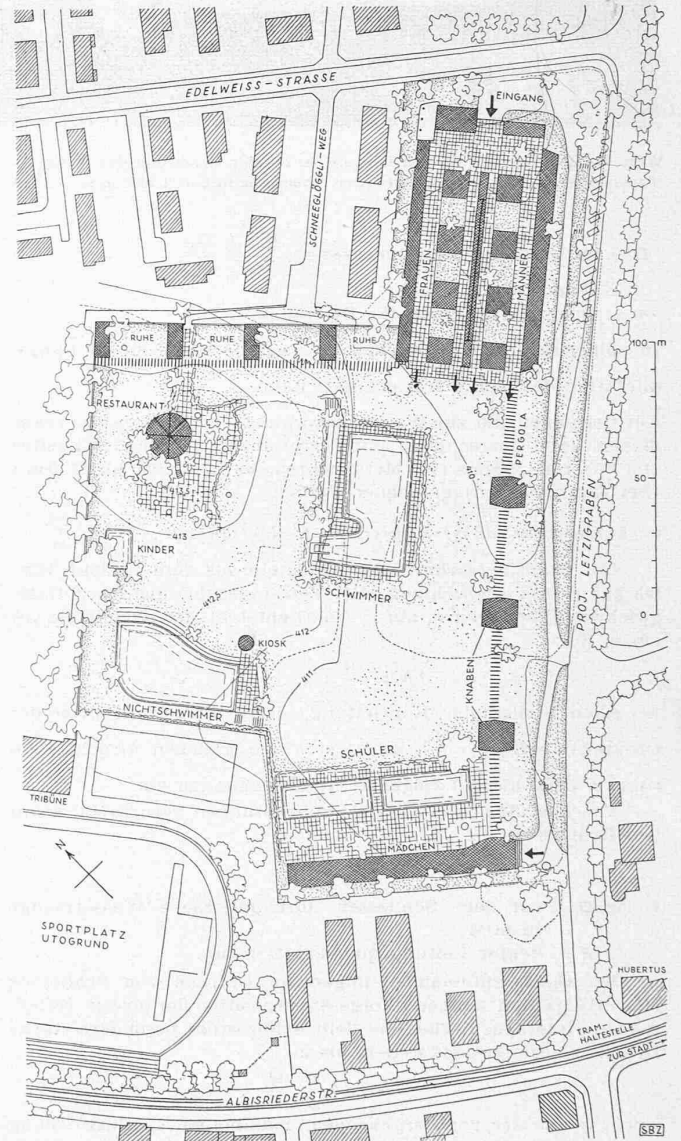
1. Preis (3000 Fr.), Entwurf Nr. 8. — Dipl. Arch. MAX FRISCH, Zürich Lageplan 1 : 2500; oben Profil NW-SO 1 : 800
