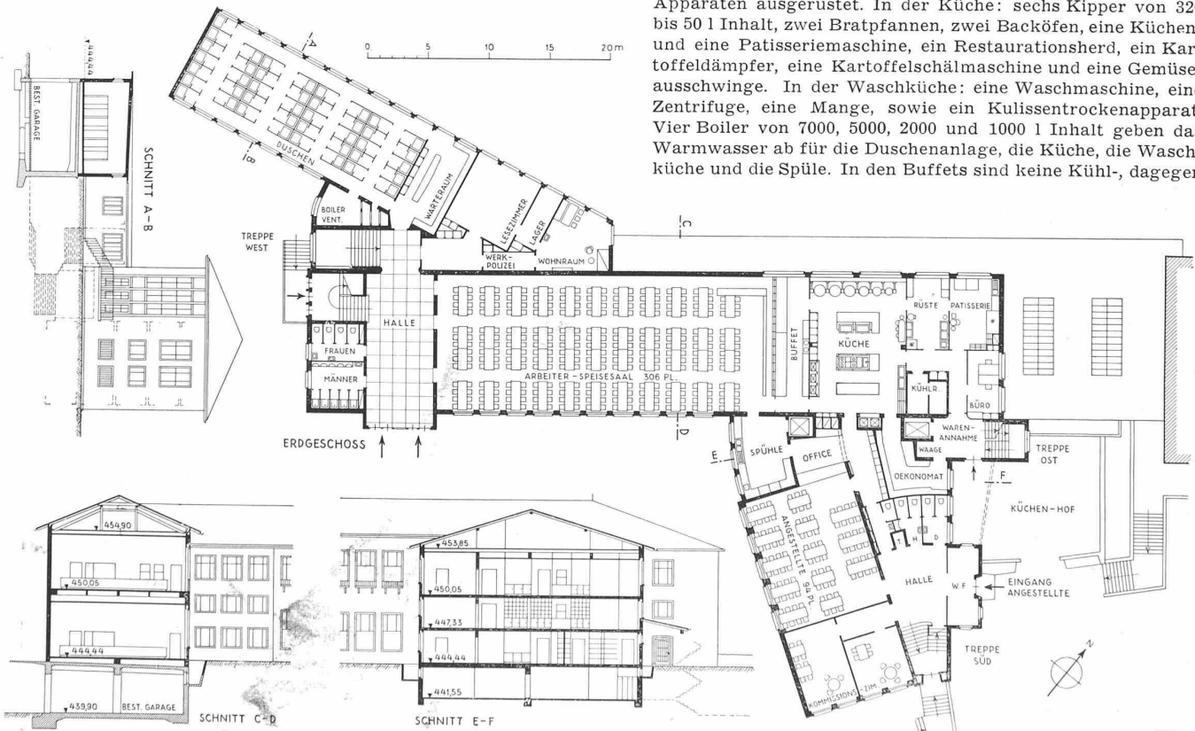
Abb. 6. Wohlfahrtshaus der Werkzeugmaschinenfabrik Bürhle & Co., Zürich-Oerlikon
