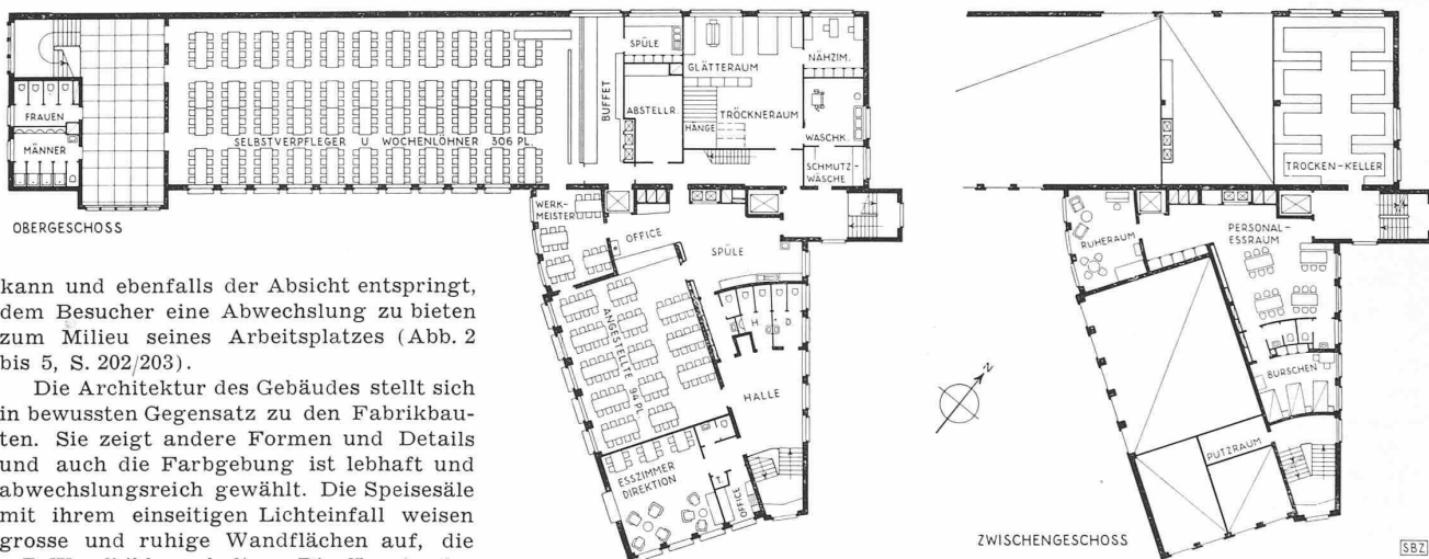
Abb. 8. Obergeschoss, rechts Zwischengeschoss. — Grundrisse 1 : 500
