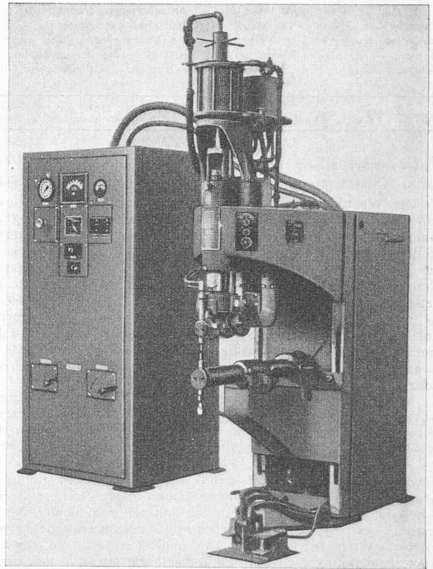
Abb. 5. Nach dem kapazitiven Aufladungsprinzip arbeitende Punktschweissmaschine mit Kondensator und Steuergerätekasten
