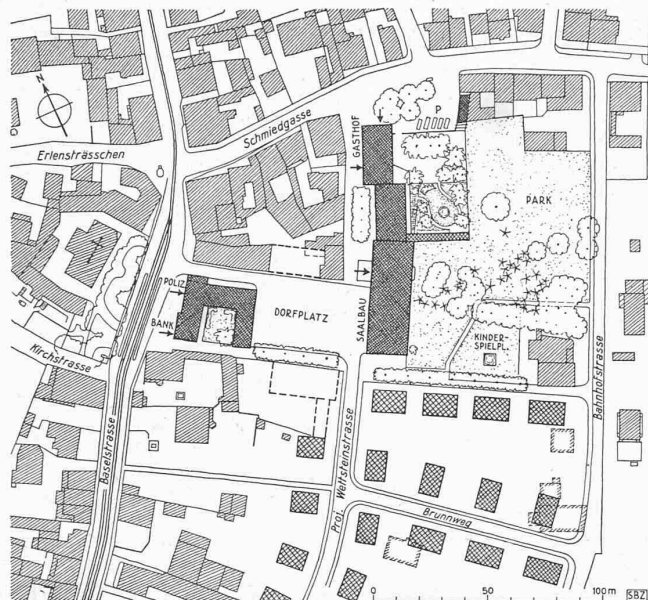
4. Preis (1700 Fr.). Entwurf Nr. 16. Verfasser Arch. FRITZ WEISS Bebauungsplan 1 : 3000 und Perspektiven
