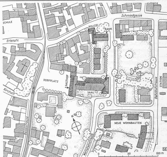
Dorfplatz Lageplan 1 : 3000
