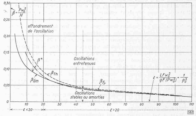
Fig. 4. Courbes \beta_{Th} = \beta(\varepsilon) Thoma, \beta_{Fr} = \beta(\varepsilon) Frank \beta^* = \beta(\varepsilon) et \beta_{lim} = \beta(\varepsilon) Région \varepsilon > 20 : validité des courbes \beta_{Fr} ou \beta^* Région \varepsilon < 20 : validité de la courbe \beta_{lim}
