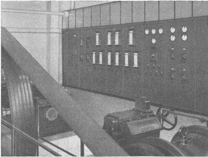
Meßtafel im Maschinenraum eines Kühlhauses
