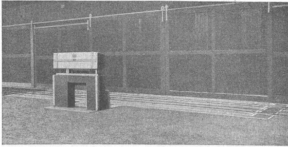
40 t Geleisewaage mit armierter Betonbrücke, torsionsfreien Hebeln und verstellbaren Schneiden.
