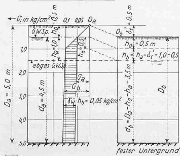
Abb. 7. Zahlenbeispiel für graphische Setzungsanalyse bei stark zusammendrückbarem Boden
