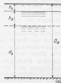
Abb. 6. Schichtverhältnis für das Zahlenbeispiel
