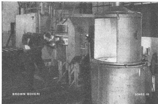
Härteöfen für hochlegierte Werkzeugstähle: Elektroden-Salzbadofen bis 1350° C (im Bild vorn) und Doppelkammerofen (hinten) mit metallischen Widerständen bis max. 1250° C.
