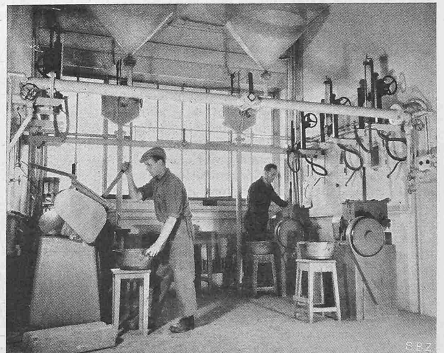
Abb. 6. Kneterei
