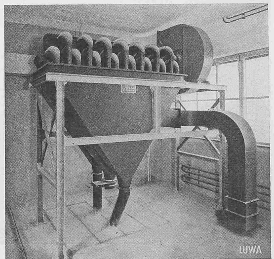
Abb. 1. Parallelgeschaltete Kleinzyklone
