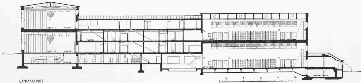
LÄNGSSCHNITT
