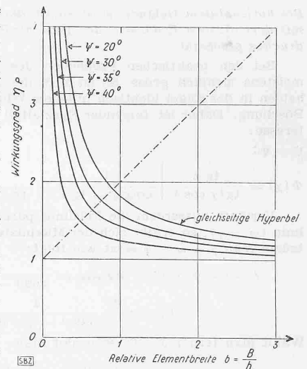
Abb. 10. Theoretischer Wirkungsgrad von Elementen
