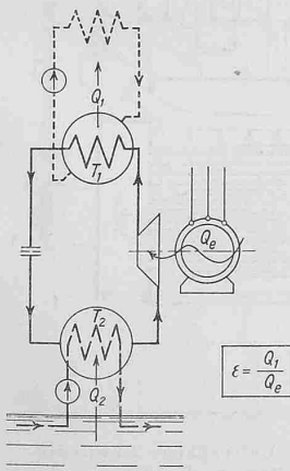
Abb. 2. Schema einer Wärmepumpanlage
