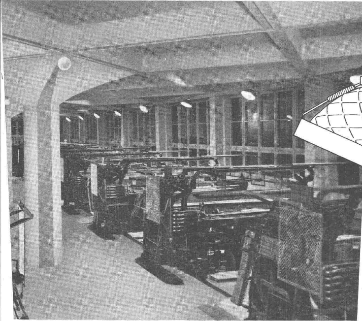
Beleuchtung des Websaales einer Tuchfabrik
