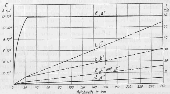
Abb. 6. Vergleich von Energieaufwand E und Flugzeit t der V2 mit zwei modernen Flugzeugen
