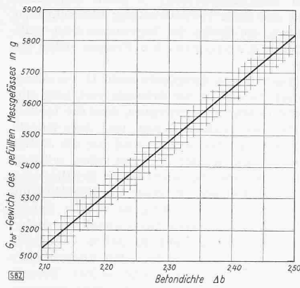
Abb. 1. Bestimmung der Betondichte aus dem Gewicht des gefüllten Messgefässes. Sonderfall für: Rauminhalt des Messgefässes V_m = 2052 \text{ m}^3 Gewicht „ „ G_m = 1202 \text{ g} Gewicht des zusätzlichen Wassers W_z = 320 \text{ g}
