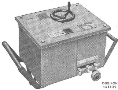
Schweisstransformator Typ EST-K 175 für max. 175 A, mit stufenloser Schweißstrom-Regulierung
