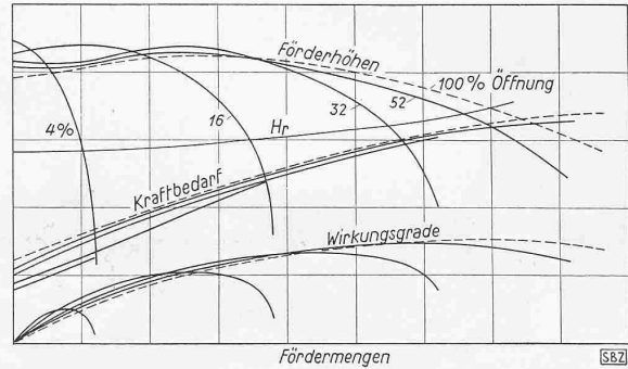
Abb. 5. Regelung durch drehbare Leitschaukeln; Förderhöhen-, Kraftbedarfs- und Wirkungsgradkurven für verschiedene Öffnungsstellungen der Leitschaukeln
