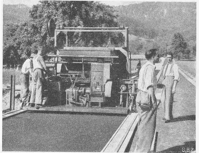
Abb. 1. Einbau eines 3 cm starken Teerasphalt-Betons (Sparbelag) in Langnau am Albis mit Strassenfertiger Racowaldvogel, im Sommer 1944 durch die Firma Gebr. Krämer, Zürich
