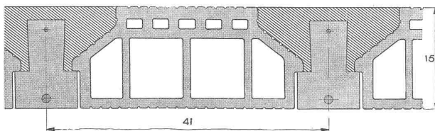
Decken-Querschnitt bei Verwendung der zementsparenden Spezial-Deckensteine
