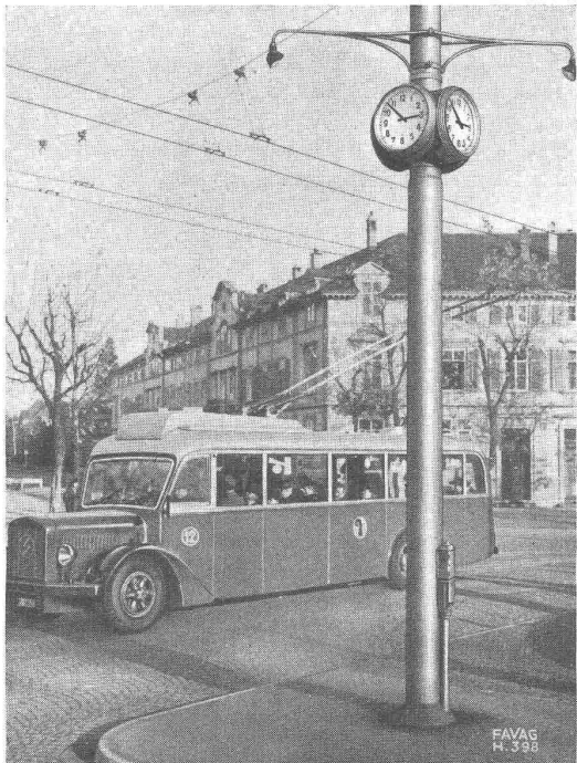
Horloge à quatre faces de Ø 60 cm d'un grand réseau urbain comprenant plus de 1000 horloges secondaires, commandées par une centrale horaire de 20 lignes.
