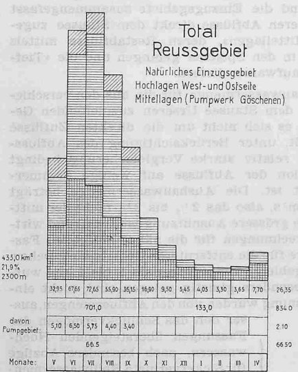
Abb. 3. Abflussmengen der ausgenützten Einzugsgebiete
