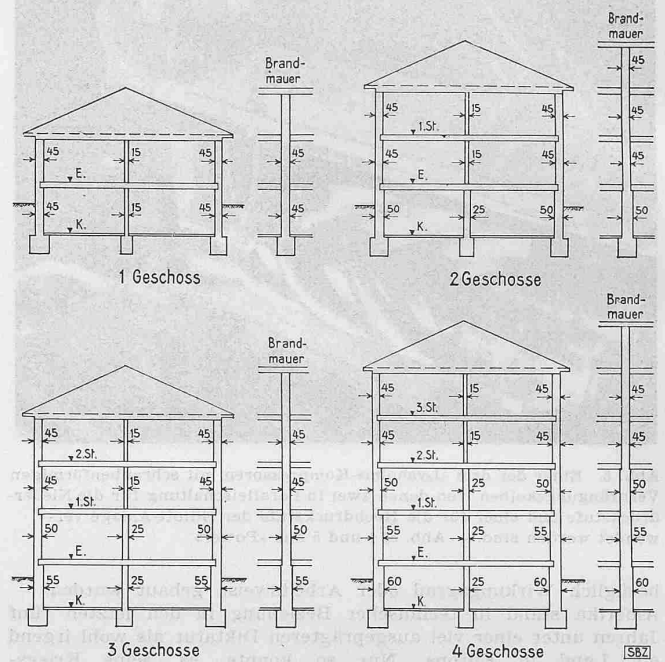
Abb. 2. Bruchstein-Mauerwerk für Aussenwände und Brandmauern mit wenigstens 600 kg/cm 2 Steifigkeit. Die Zwischenmauern sind in Formsteinmauerwerk vorgesehen
