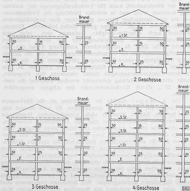
Abb. 5. Formstein-Mauerwerk (Ziegel-, Zement-, Kalksandstein) mit wenigstens 160 bis 200 kg/cm 2 Steifigkeit nach 28 Tagen. Für das aufgehende Fassadenmauerwerk sind Spezialsteine zu verwenden
