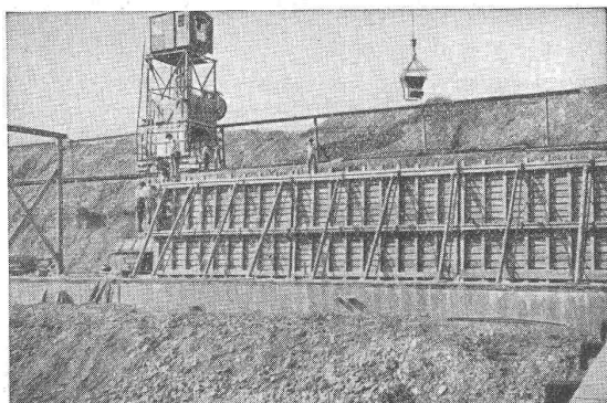
Schalung einer Quaimauer, Rheinhafen in Basel (Gebr. Stamm, Basel)
