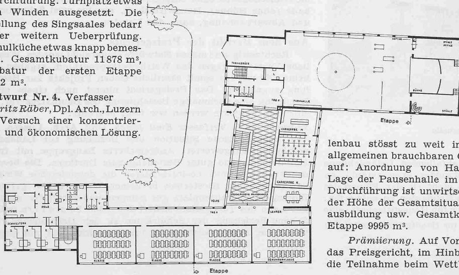
Obergeschoss, darunter Erdgeschoss 1 : 600 und Perspektive
