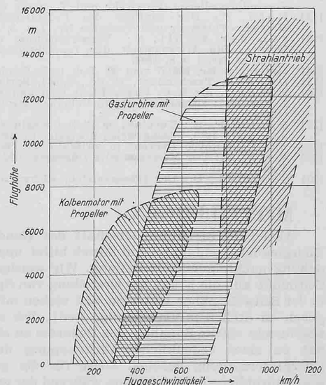
Abb. 38 (rechts). Geschwindigkeitsbereiche und Höhenlagen, in denen die drei Antriebsarten voraussichtlich als geeignet erscheinen. (Aus Bd. 126, S. 115)
