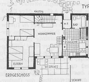
ERDGESCHOSS
