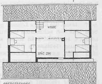
OBERGESCHOSS
