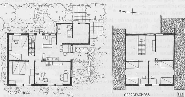
Typ B, 1 : 300
