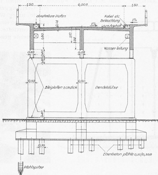
Bild 13. Brücken-Zufahrt
