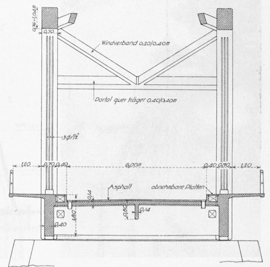
Bild 14. Hauptöffnung
