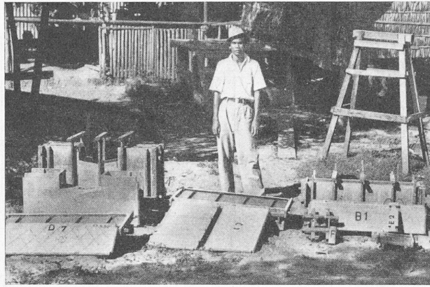
Bild 15. Mörtelplatten für die Einschalung der Zugbänder
