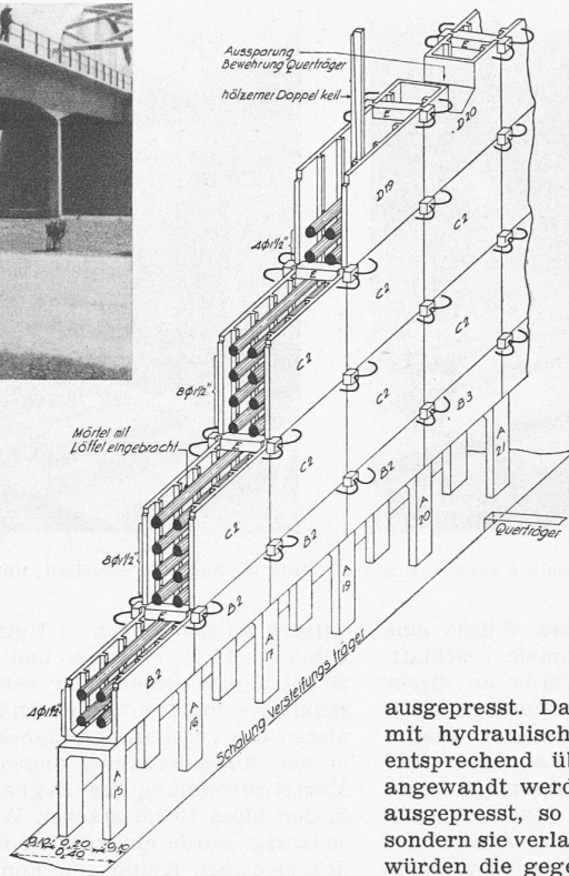
Bild 23. Verschaltung des Zugbandes mit Mörtelplatten
