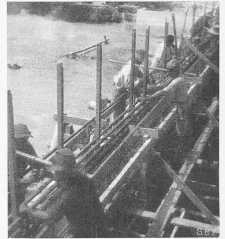
Bild 16. Verlegen der Zugbandeisen
