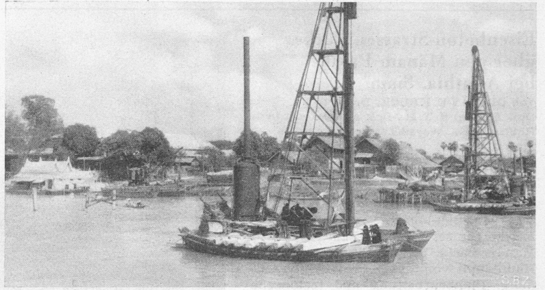
Bild 5. Rammern eines Holzpfeils (vorn) und eines Eisenbetonpfeils (hinten)
