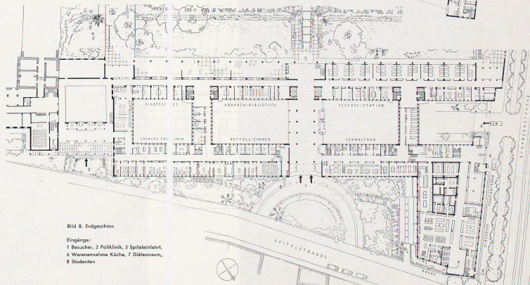
BÜRGERSPITAL BASEL Grundrisse und Schnitte Masstab 1:800
