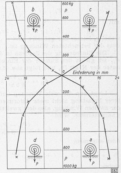
Bild 6. Gemessene Federdiagramme, x = Berechnete Knickpunkte
