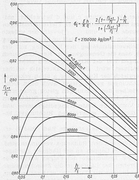
Kurven zum schnittweisen Entwurf von Spiralfedern Bild 4. Beginn bei der äussersten Windung
