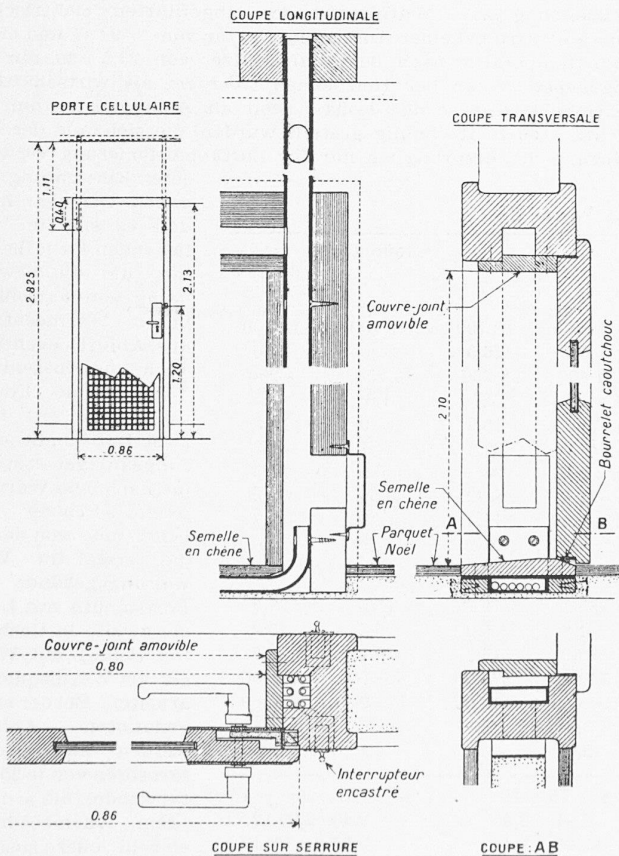
Bild 1. Französischer Türblock
