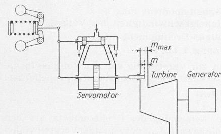
Bild 1 bis 3. Schematische Gegenüberstellung der Drehzahlreglung von Turbinen u. Flugzeug-Triebwerken
