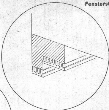
Fensterstürze
