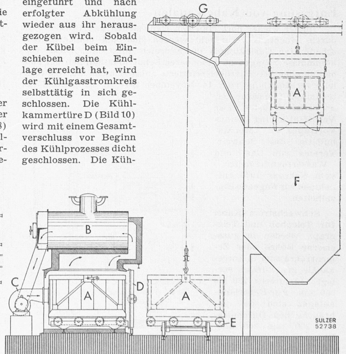
Bild 10. Sulzer-Kokskühlanlage nach dem Kammertyp. Schematischer Querschnitt. A Kokskübel, B Dampfkessel, C Gebläse, D Kühlkammertüre, E Kübelwagen, F Kokssilo, G Fahrkran
