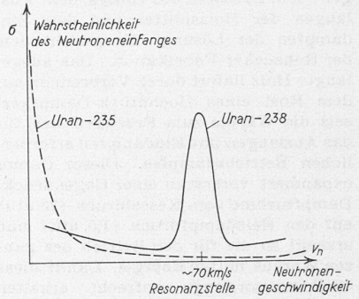
Bild 15. Die Einfangungswahrscheinlichkeit für Neutronen verschiedener Geschwindigkeiten in Uran-235 und Uran-238
